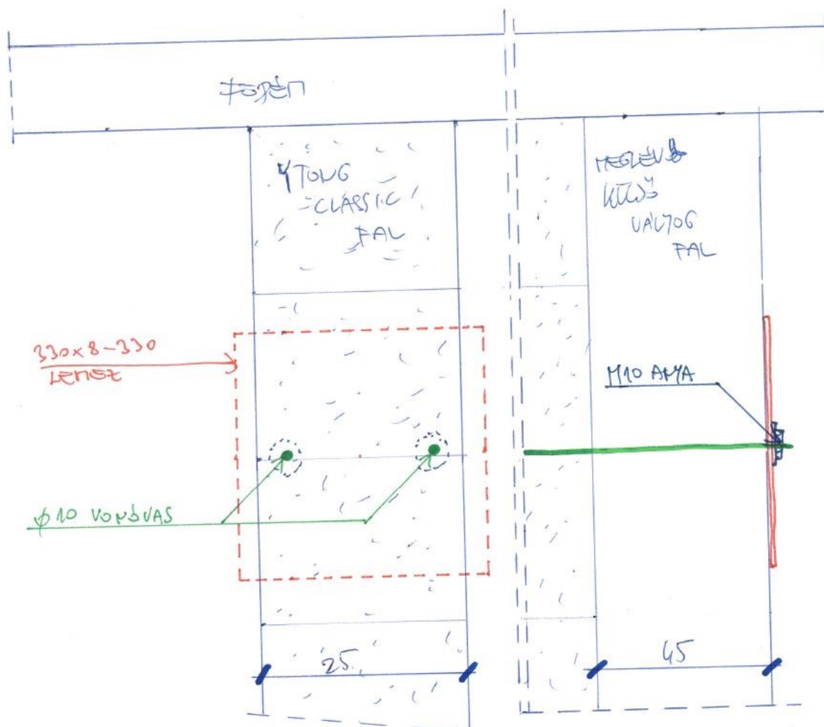
8. ábra: Vonóvasak vezetése, lehorgonyozása
