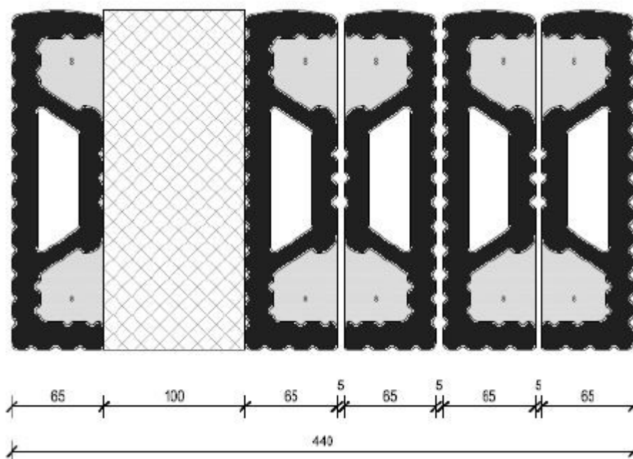
7. ábra: Elemmagas áthidalók beépítése
